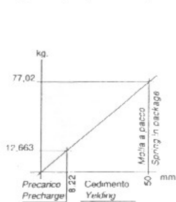
MOLLA INFERIORE LOWER SPRING
